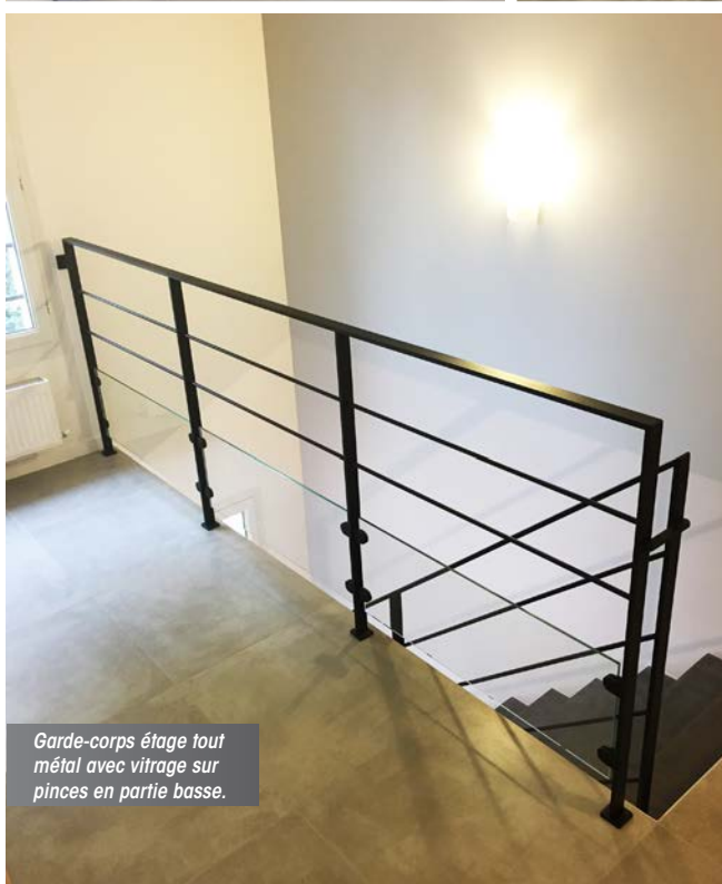
Garde-corps étage avec poteaux et lisses acier vitrage sur pinces en partie basse et main courante bois.
